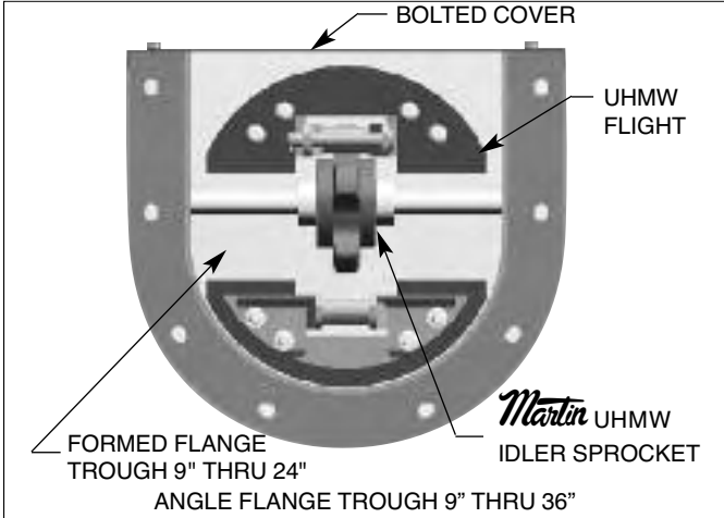
Idler Return
