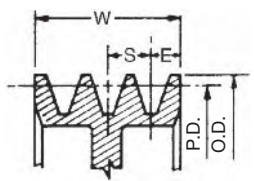
Groove Dimensions
